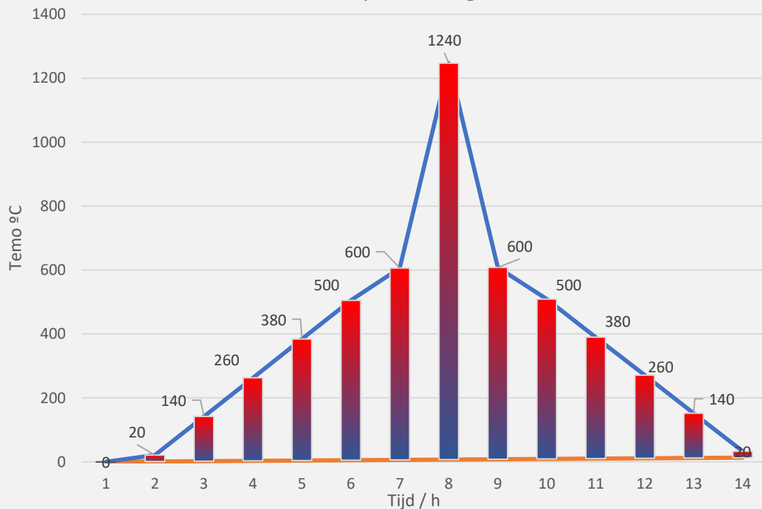
Biscuit met 120°C p/h steengoed 1240°C
